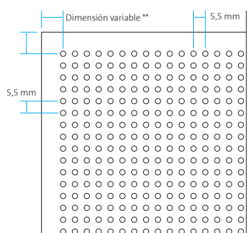
Perforación \varnothing 2,5 mm Área perforada ~ 16%
