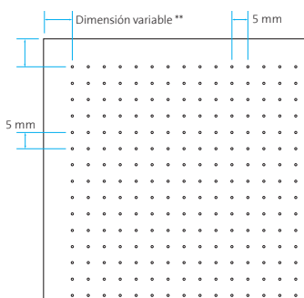
Perforación ultra-micro \varnothing 0,7 mm Área perforada ~ 1,5%
