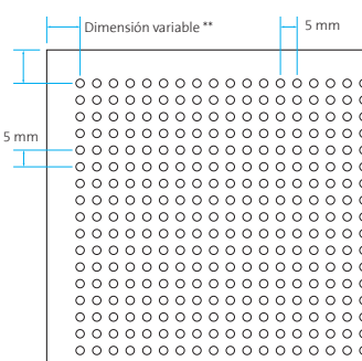
Perforación \varnothing 2,5 mm Área perforada ~ 20%
