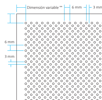
Perforación \varnothing 2 mm Área perforada ~ 18%
