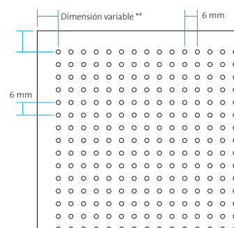
Perforación \varnothing 2 mm Área perforada ~ 9%
