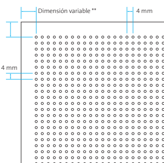
Perforación \varnothing 1,5 mm Área perforada ~ 11%
