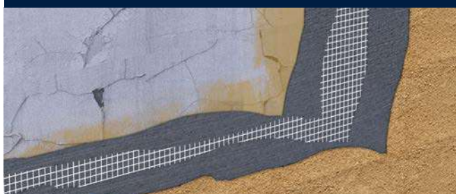
SISTEMA RFCH5
